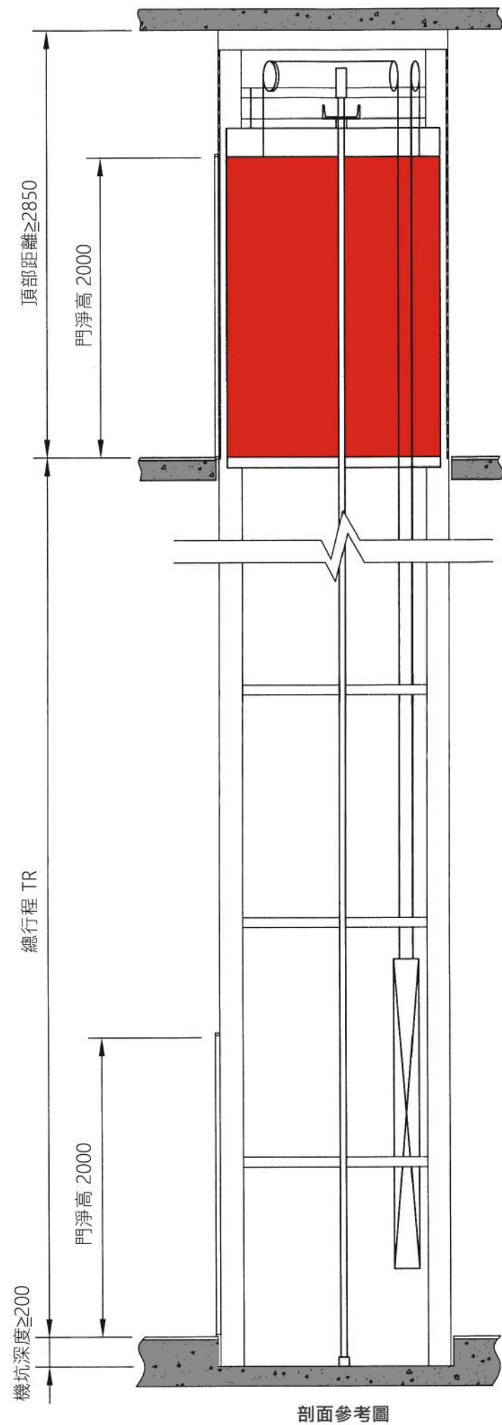
剖面參考圖
